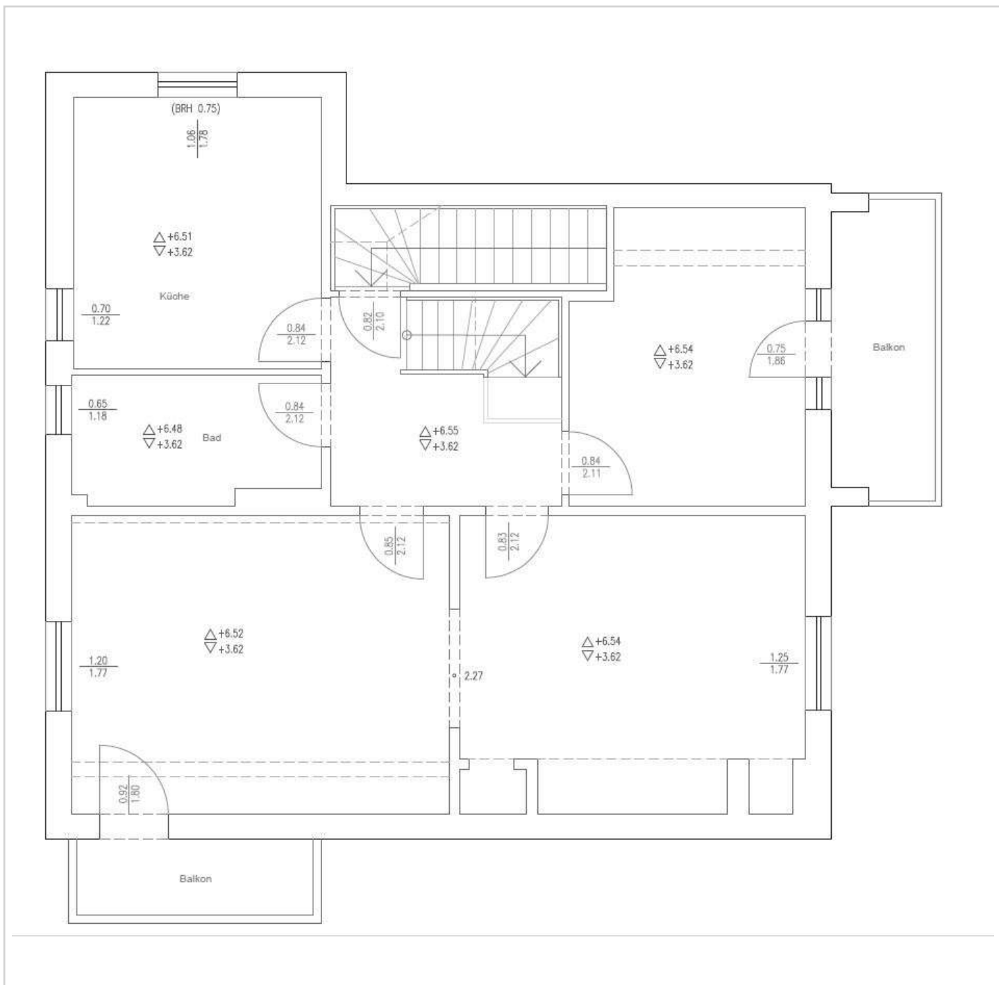
Grundriss Obergeschoss
